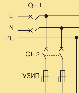
Однофазная система
