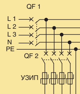
Трехфазная система
